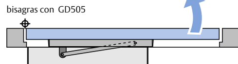
OBM505 montado en cara bisagras con GD505
