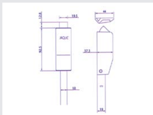
Detalle carcasa
