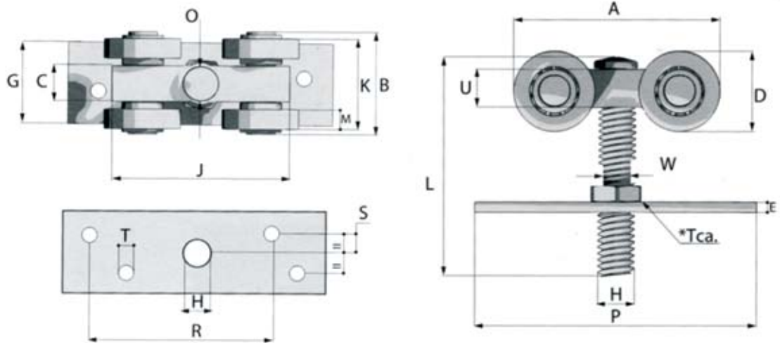
CARRO 4 RUEDAS
