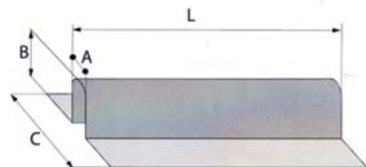
Riel inferior para rueda de perfil redondo
