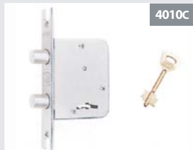
CERROJO DE EMBUTIR REFORZADO PARA PUERTA EXTERIOR DE CRISTAL DE SEGURIDAD
